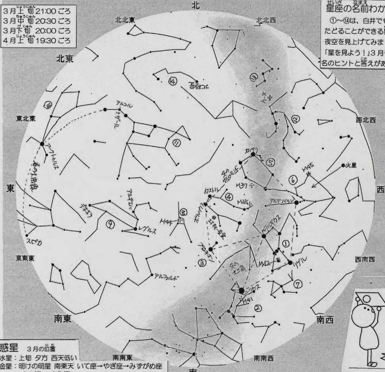
見たい方向(例えば南)を向き、この図を頭の上にかざす。方位をあわせ、星を見つける。
