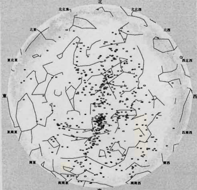
星図 ステナナビゲーターVer.5/(株)アストロアーツ/(株)アスキー 下図 国立天文台
